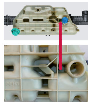
Figure 2 : Vase d'expansion avec moulures et orifices d'écoulement.
