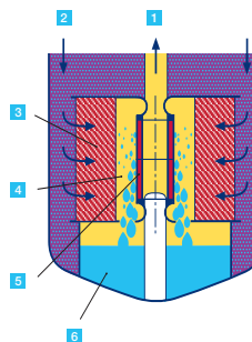
Diagrama de un filtro de dos etapas con separador de agua integrado
