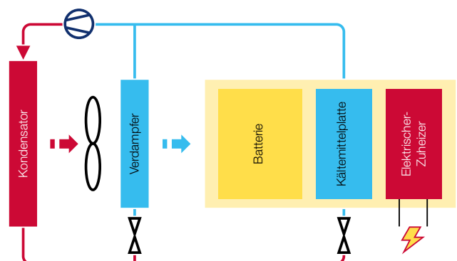
Kältemittelbasierender Kreislauf
