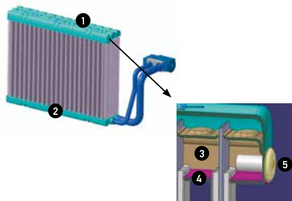
Schematische Darstellung – Speicherverdampfer: (1) Verdampferblock mit 40 mm Tiefe, (2) Speicherblock 15 mm Tiefe, (3) Kältemittel, (4) Latentmedium, (5) Blindniet
